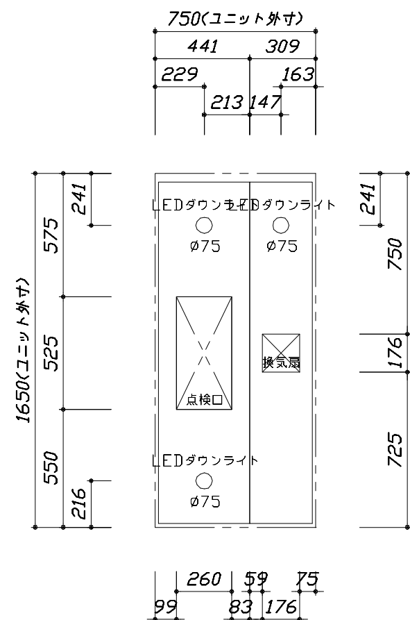
< 天井伏図 >
