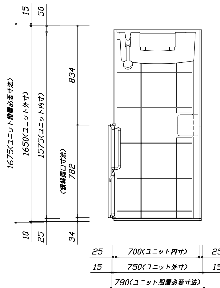
< 平面図 >
