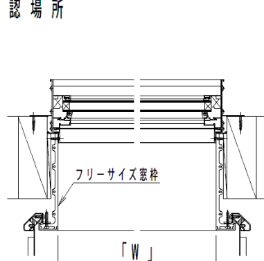
窓サッシ納まり図(横断面)
