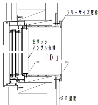
窓サッシ納まり図(縦断面)
