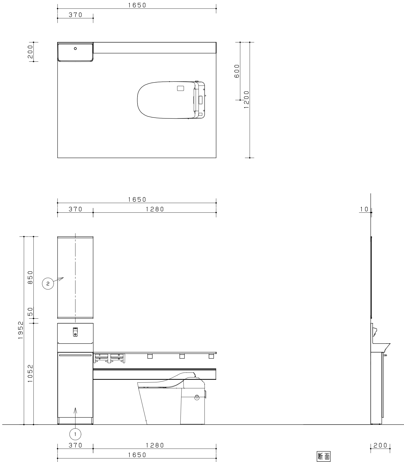
展開図
